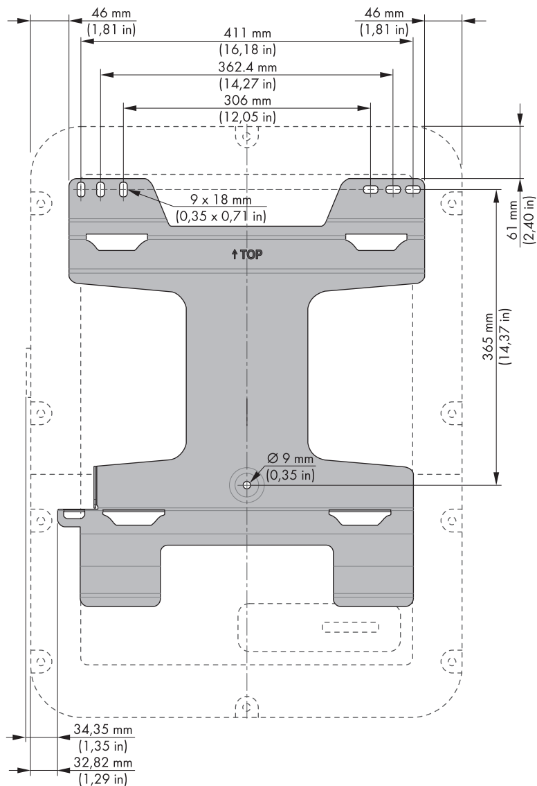
Imagen 18 : Posición de los puntos de fijación
