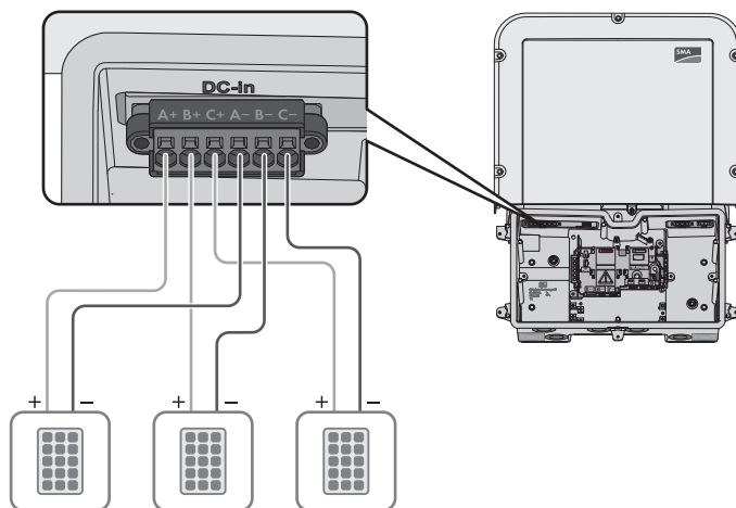
Imagen 24 : Vista general de la conexión en el funcionamiento normal
