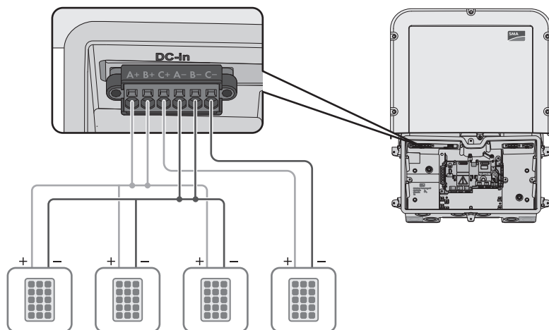
Figure 40 : Vue d'ensemble du raccordement pour « 4-String-Operation »
