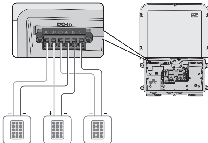
Figure 39 : Vue d'ensemble du raccordement en fonctionnement normal
