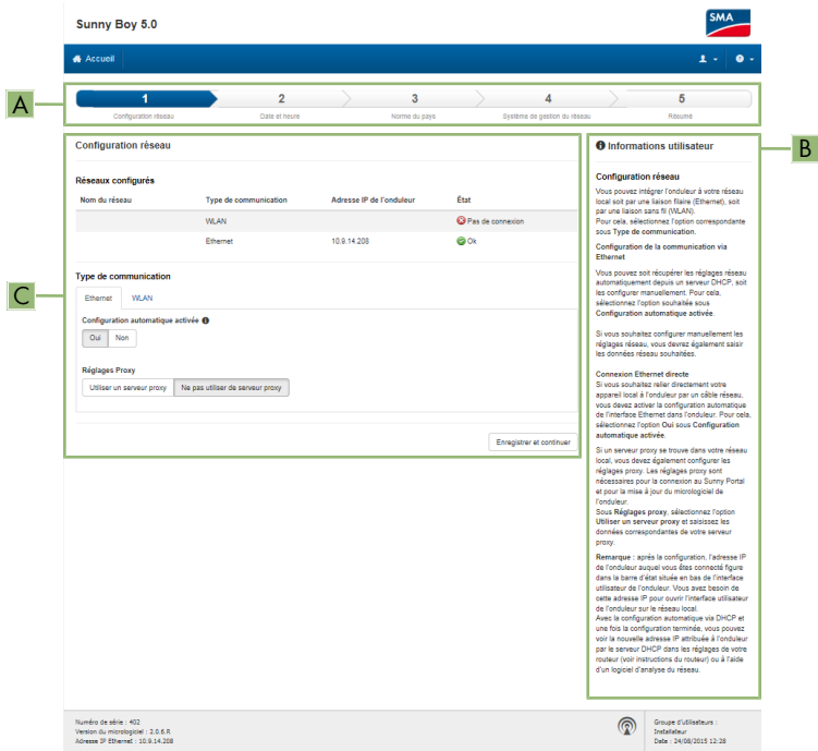
Figure 45 : Composition de l’assistant d’installation
