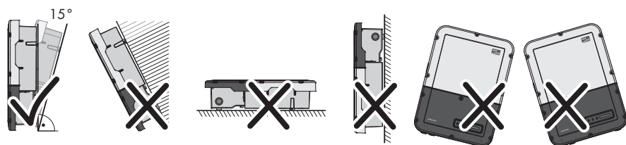
Imagen 20 : Posiciones de montaje permitidas y no permitidas
