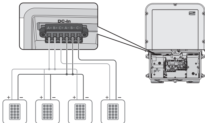
Imagen 25 : Vista general de la conexión en la "Operación de cuatro strings"
