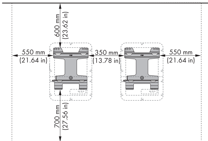
Figure 34 : Distances recommandées
