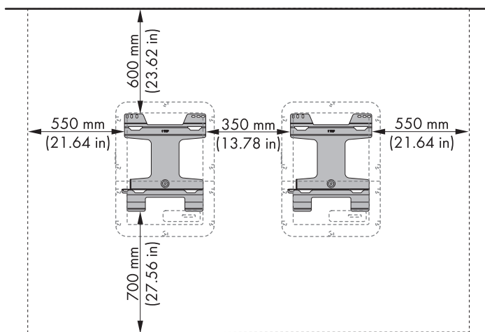
Imagen 19 : Distancias recomendadas
