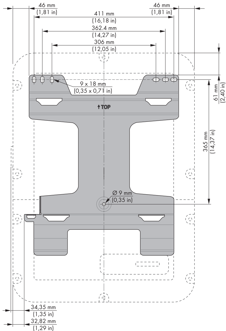
Figure 33 : Position des points de fixation
