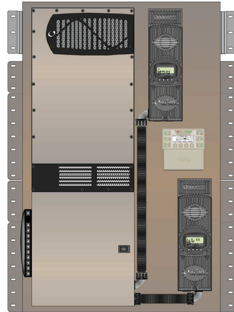
FLEXpower Radian FPR-8048A
